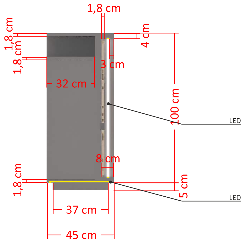
Przekrój
